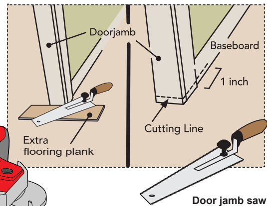
Door jamb saw
