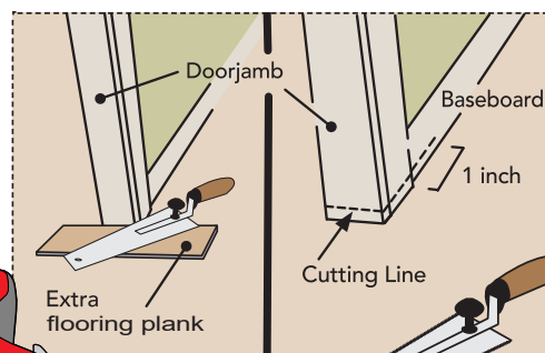
Door jamb saw
